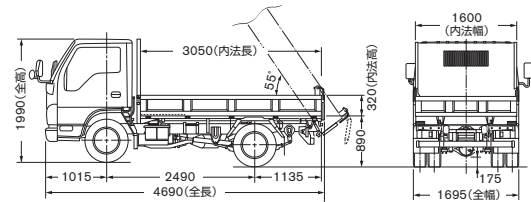
■標準幅キャブ・標準ボディ・三方開・前後固定柱無【フルスーパーロー】
