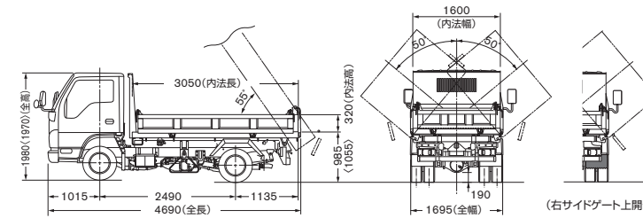
■標準幅キャブ・標準ボディ・強化型・三方開 (HD05) ・右側上開き仕様 (HD21) ・固定柱付 [高床ダブルタイヤ]
