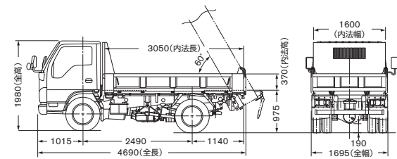
■標準幅キャブ・標準ボディ・スーパー強化型・三方開・固定柱付 [高床ダブルタイヤ]
