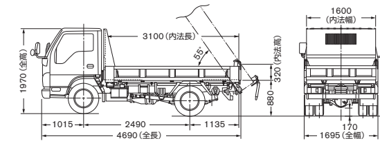
標準幅キャブ・標準ボディ・三方開・リヤ固定柱付(HD08)・無(HD09)[フルスーパーロー]
