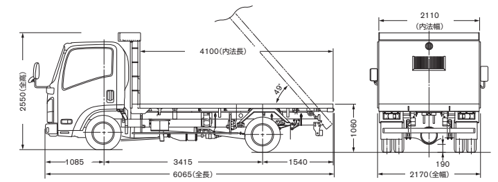
■ワイド幅キャブ・ロングボディ・フラットデッキ(*1)・固定柱無【フルスーパーロー】
