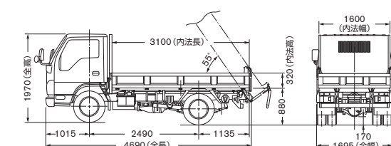
標準幅キャブ・標準ボディ・三方開・前後固定柱無[フルスーパーロー]
