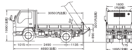
■標準幅キャブ・標準ボディ・強化型・三方開・固定柱無【フルスーパーロー】
